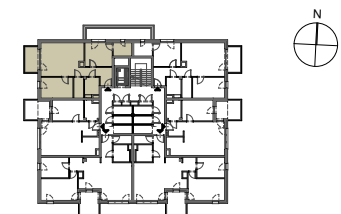
PLAN BUDYNKU C POZIOM 1
