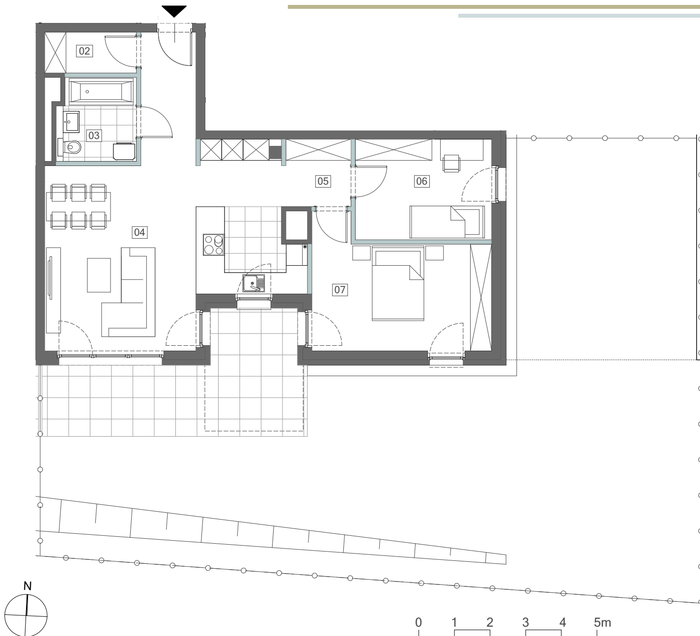
PLAN BUDYNKU C POZIOM 0
