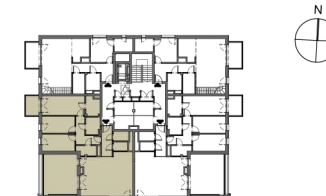
PLAN BUDYNKU A POZIOM 3
